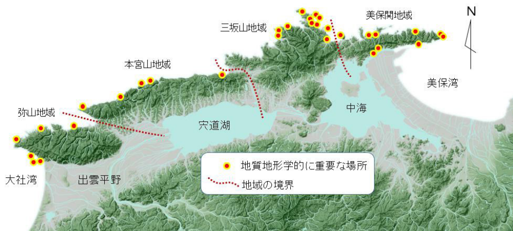
図1 島根半島の地形の特徴と地質学的に重要な場所。
