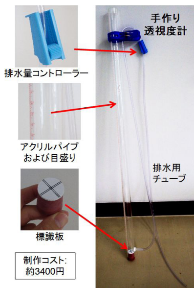
図3 本プロジェクトで作成した透視度計の特徴。
