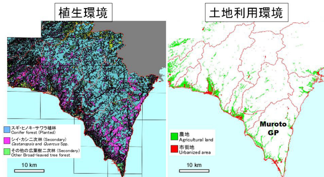
図2 室戸ジオパークおよび周辺地域の植生（左）および土地利用（右）。環境省自然環境局生物多様性センター・自然環境情報 GIS 提供システム（1/2.5万植生調査）を元に作成。
