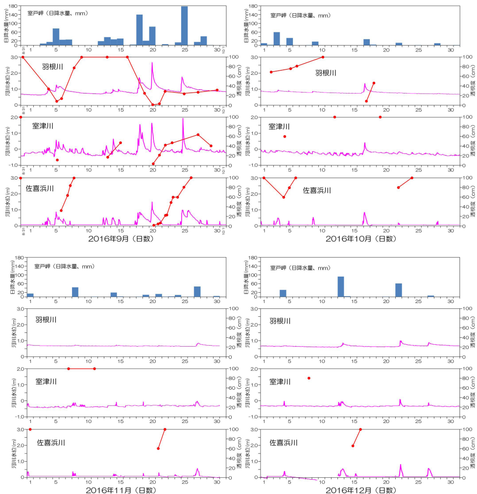
図5 室戸岬の日降水量(上段)および河川水位と透視度の変化(2016年9～12月)。室戸岬の日降水量は気象庁、河川水位の時間変化は高知県土木部河川課(高知県水防観測情報)による。
